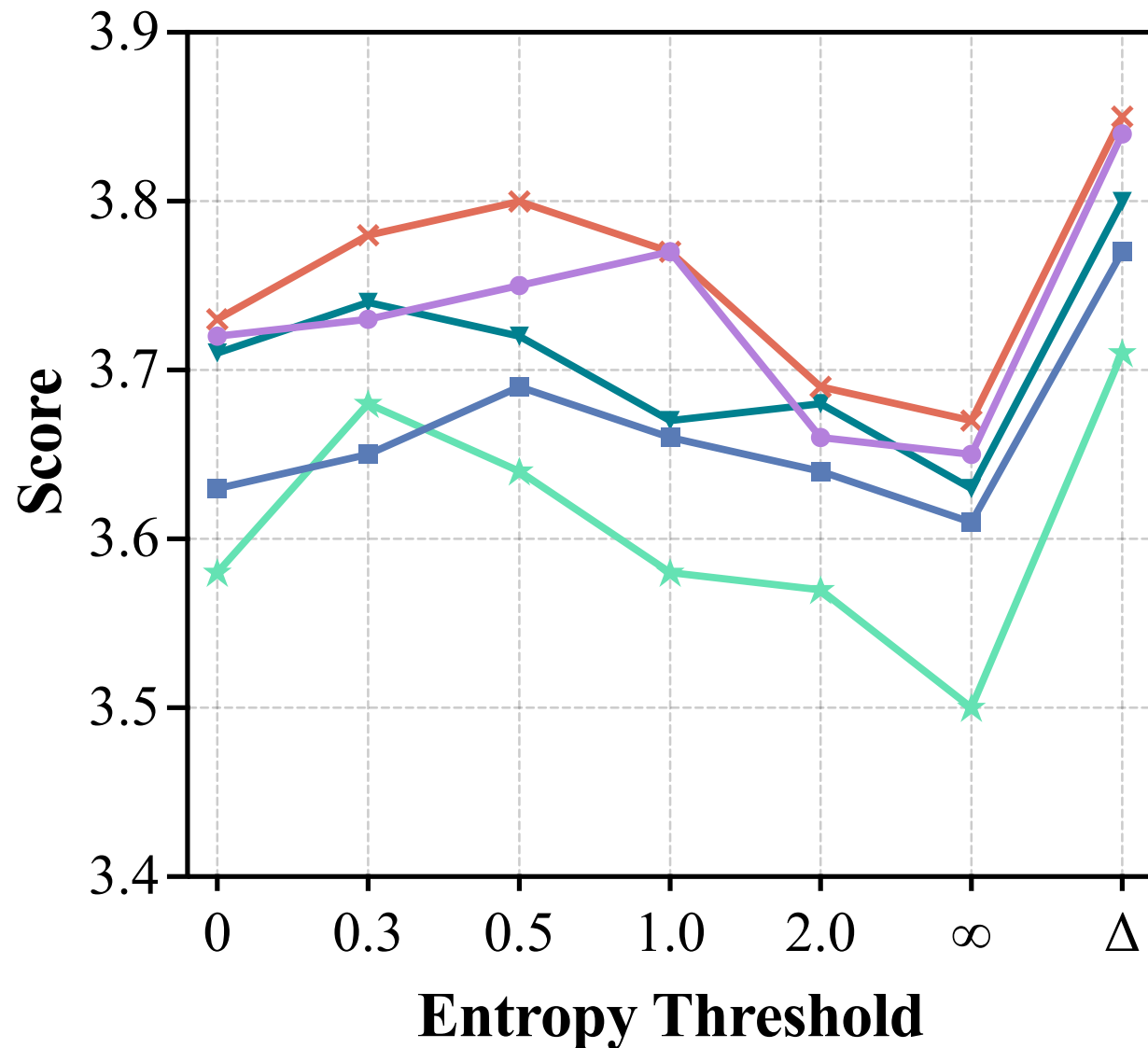
Bingo
